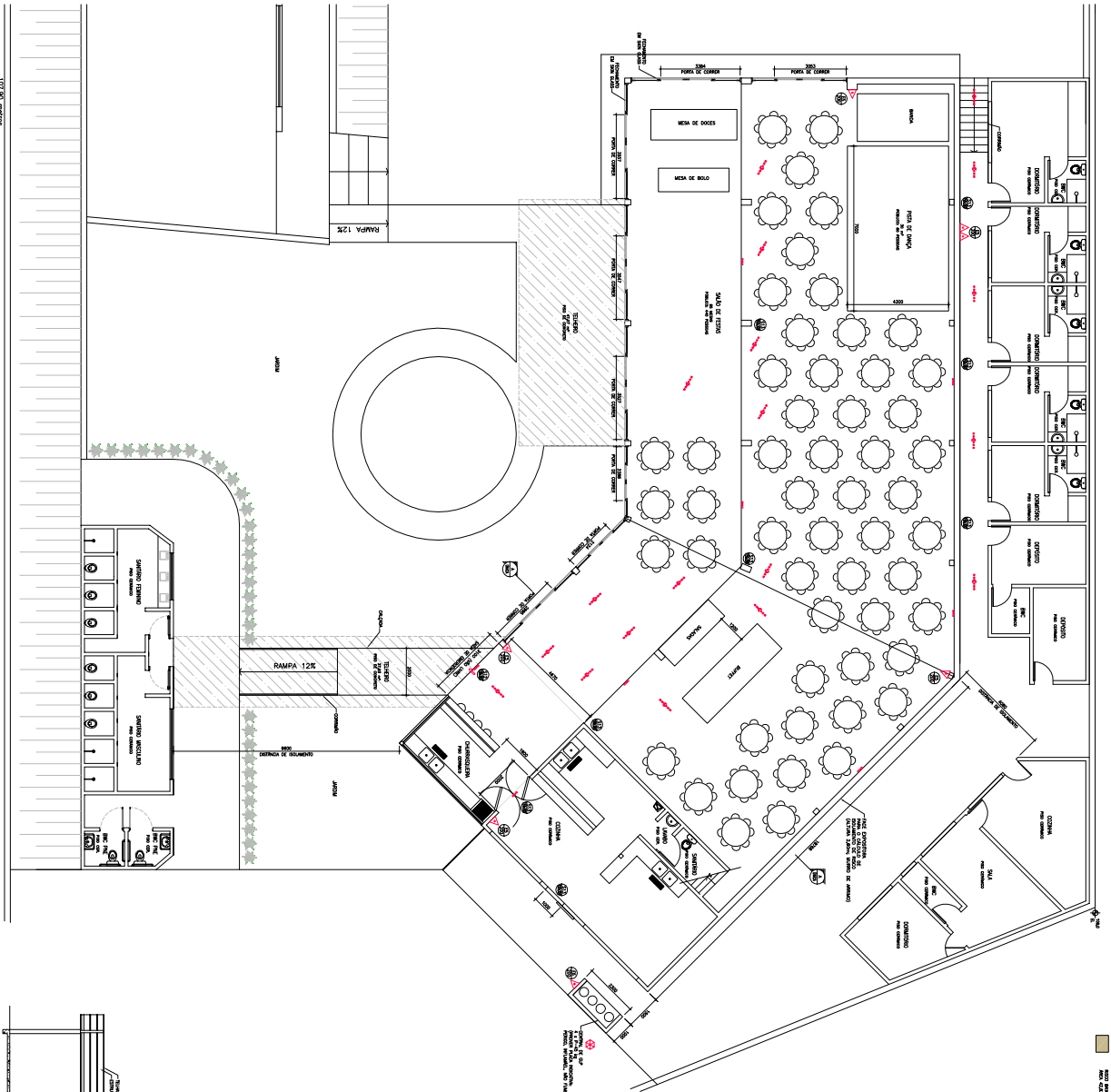
1 PLANTA BAIXA – IMPLANTAÇÃO
